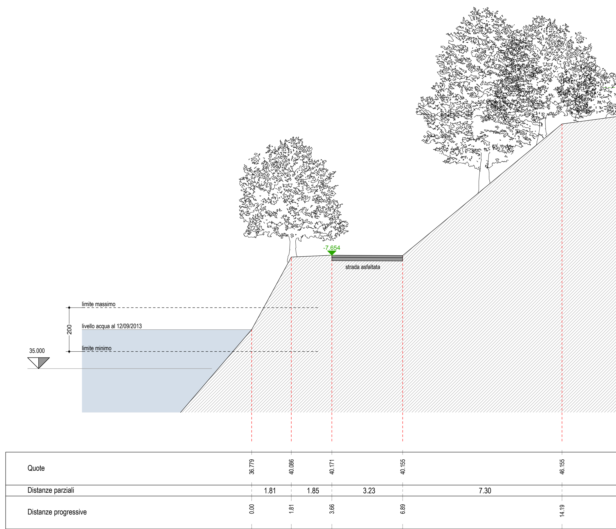
SEZIONE 1-1
